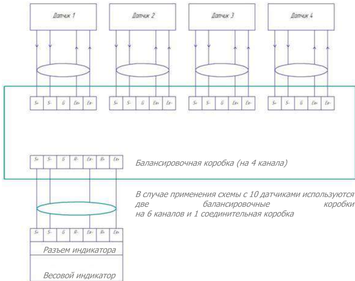
Рисунок. 2 - Схема электрических соединений весового терминала и датчиков.
