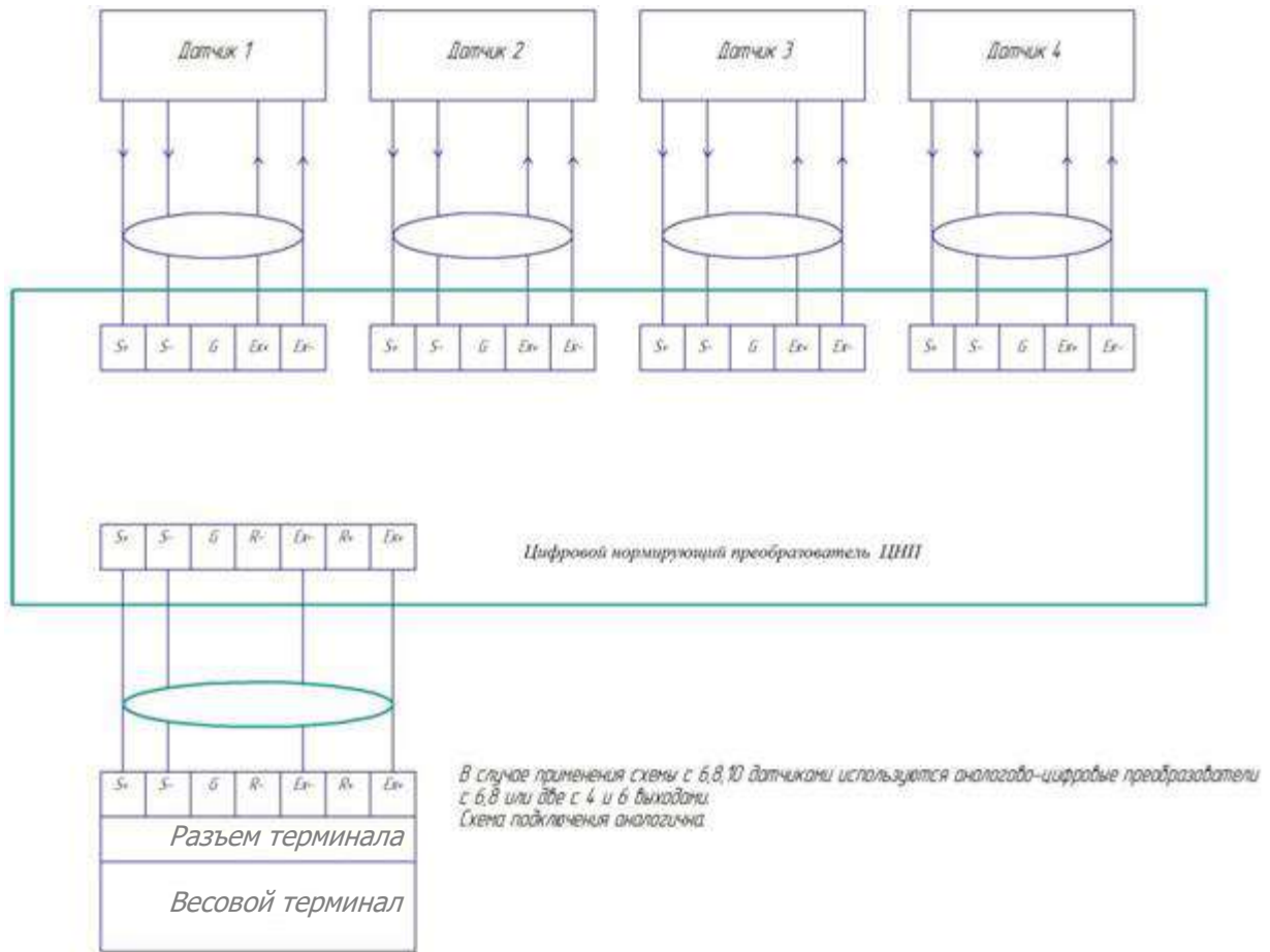
Рисунок. 1 - Схема электрических соединений весовых индикаторов и датчиков.
