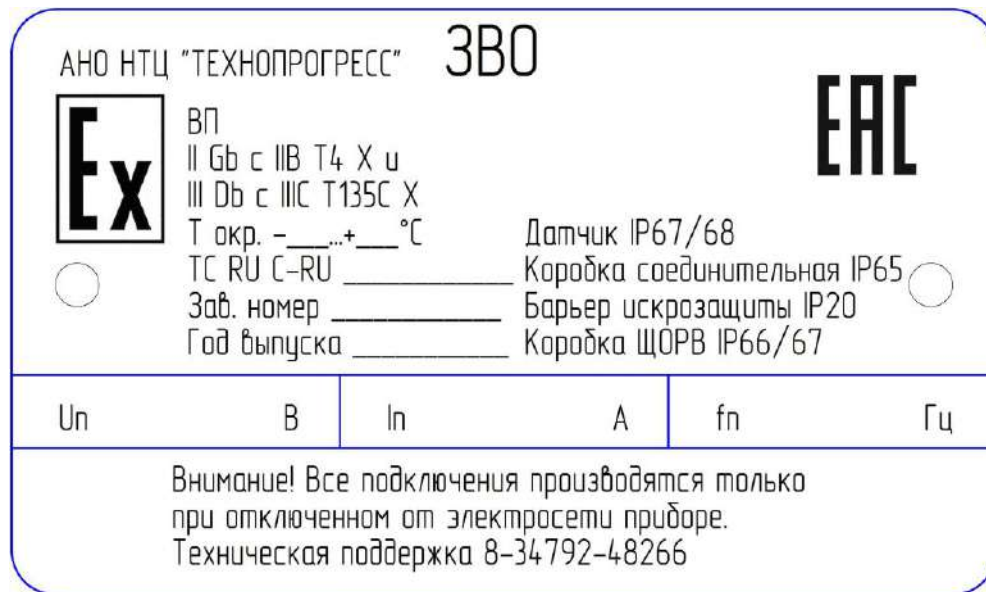
Рис. 2 Маркировочная табличка весов электронных ВП выполненных во взрывозащищенном исполнении.
